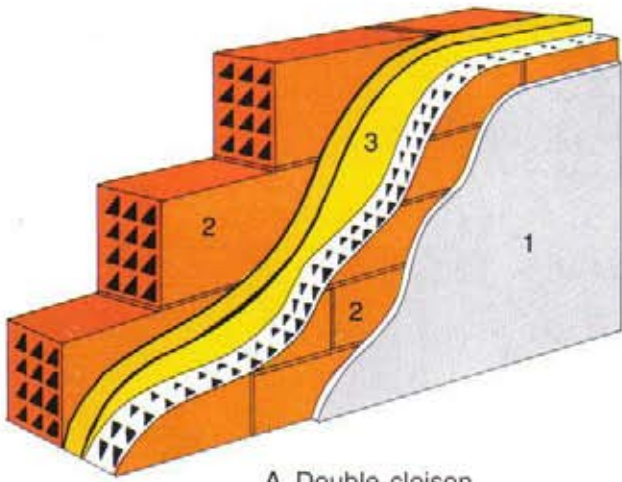
A Double cloison 1 enduit 2 briques 3 mousse de polyuréthane
