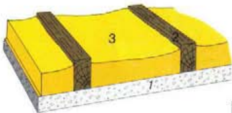
D Combes 1 plancher haut 2 poutre 3 mousse de polyuréthane
