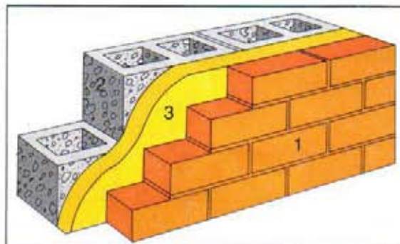
F Isolation extérieure avec parement 1 briques 2 agglos 3 mousse de polyuréthane
