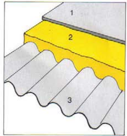
E Isolation et toiture 1 épiderme 2 mousse 3 tôle ondulée
